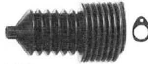
M.R.1471 fuelle cremallera asistida r.o. 7700781095
